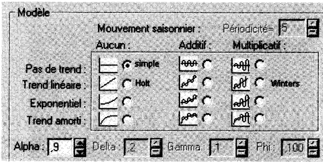
Figure 11.20. Sélection du coefficient Alpha
