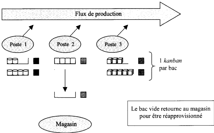
Figure 8.8. Approvisionnement par kanban simple (double bac) d'une chaîne de production
