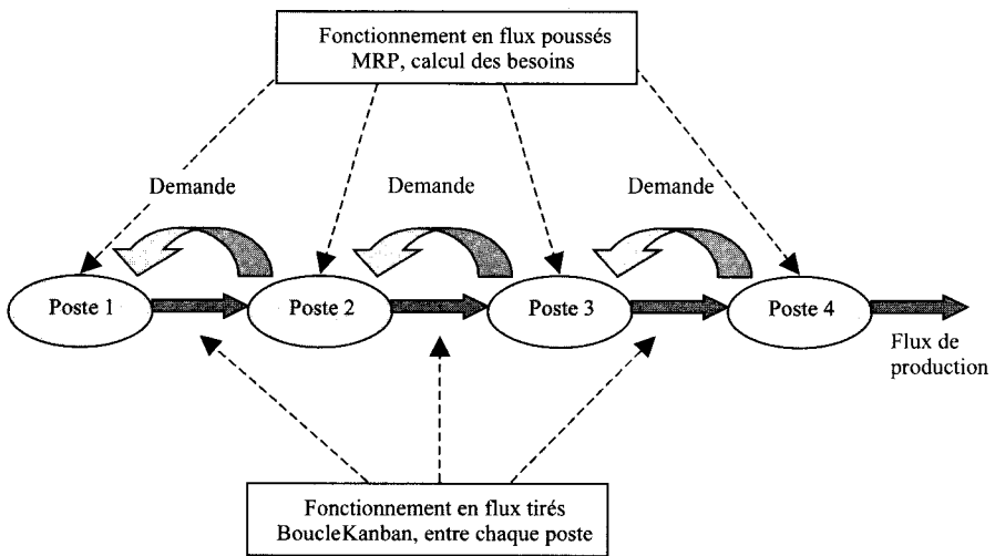
Figure 8.5. Boucles kanban entre postes de travail
