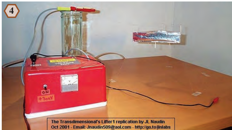
Reconstitution du « lifter » de Transdimensional Technologies par Jean-Louis Naudin . Des fils de nylon fixés sur la table empêchent le « lifter » d'aller trop haut (gracieuseté de J.-L. Naudin).
