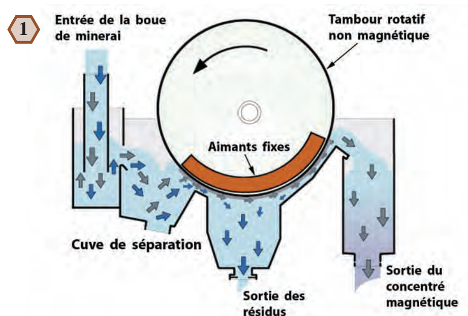
Fonctionnement d'un séparateur magnétique à tambour rotatif. Le tambour est en acier inoxydable non magnétique et les aimants sont stationnaires (courtoisie de Metso Minerals).
