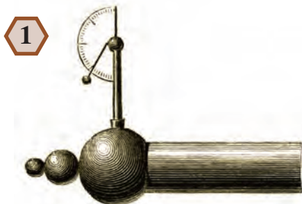
1 Électromètre de Henley installé sur le gros conducteur d'une machine électrostatique.
