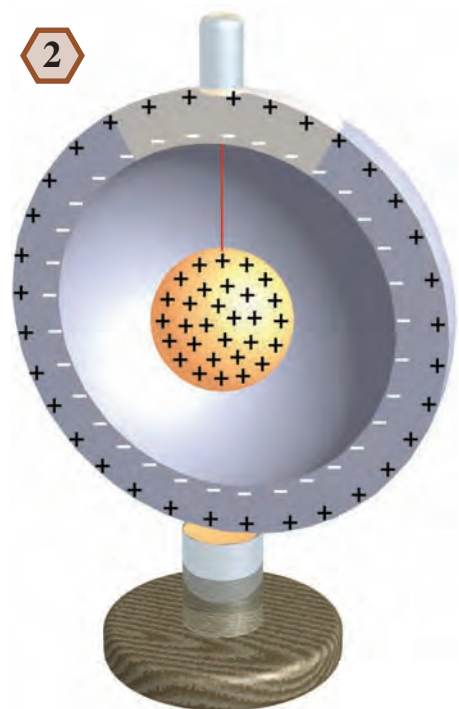
L'induction électrostatique dans la paroi d'une sphère métallique creuse, causée par une sphère chargée au centre.
