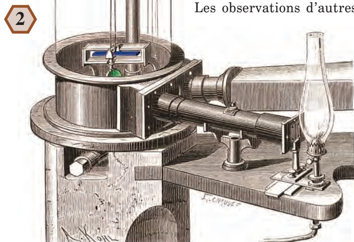
Appareil des années 1870 conçu pour mesurer et enregistrer les variations de la déclinaison magnétique.
