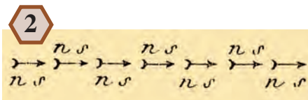
Illustration du modèle moléculaire magnétique de Coulomb (tirée de son mémoire de 1789). Les molécules magnétiques sont représentées par des petites flèches.
