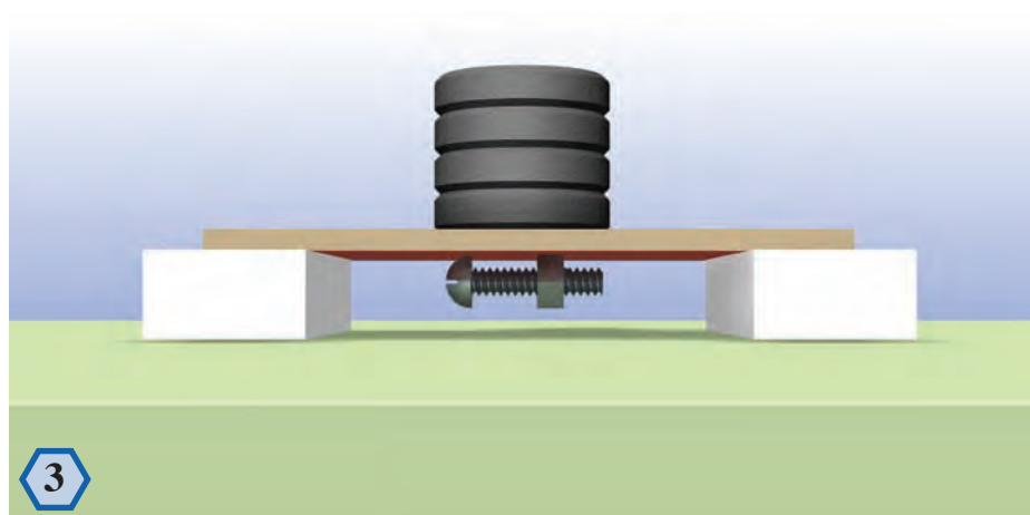
3 La force d'attraction de l'aimant traverse le carton et fait coller la vis à sa surface inférieure. Il en est de même pour les autres matériaux, sauf pour le fer.
