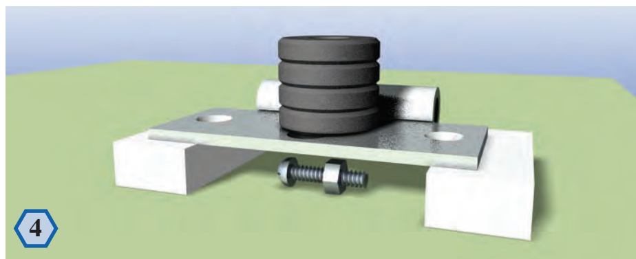
4 Une plaque de fer (battant de peinture de porte) détourne les forces magnétiques de l'aimant vers ses bords et empêche l'attraction de la vis sous la plaque.
