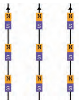
Alignement des molécules magnétiques suivant les lignes du champ magnétique d'un aimant externe. Les flèches indiquent la direction de la force sur les pôles Nord.
