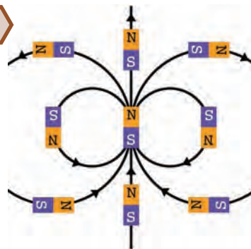
Le champ magnétique d'une molécule (celle du centre) et l'alignement des molécules voisines suivant ce champ.
