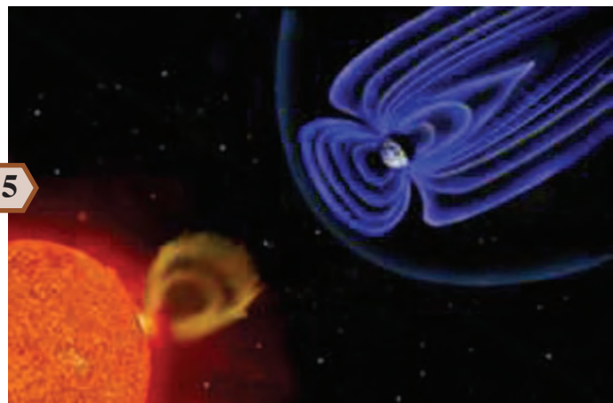
Les lignes du champ magnétique terrestre sont modifiées et rendues asymétriques sous l'influence du vent solaire (illustration de Steele Hill – SOHO/NASA).
