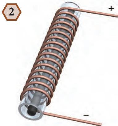
Aimantation d'une tige d'acier par un courant solénoïdal issu d'une pile électrique, non visible sur la figure. Le tube de verre permet d'isoler le fil de cuivre de la tige d'acier.
