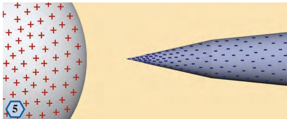
Un objet chargé d'électricité positive (à gauche) induit des charges négatives sur une pointe métallique dans son voisinage. La densité des charges électriques est d'autant plus grande qu'on approche du sommet de la pointe.
