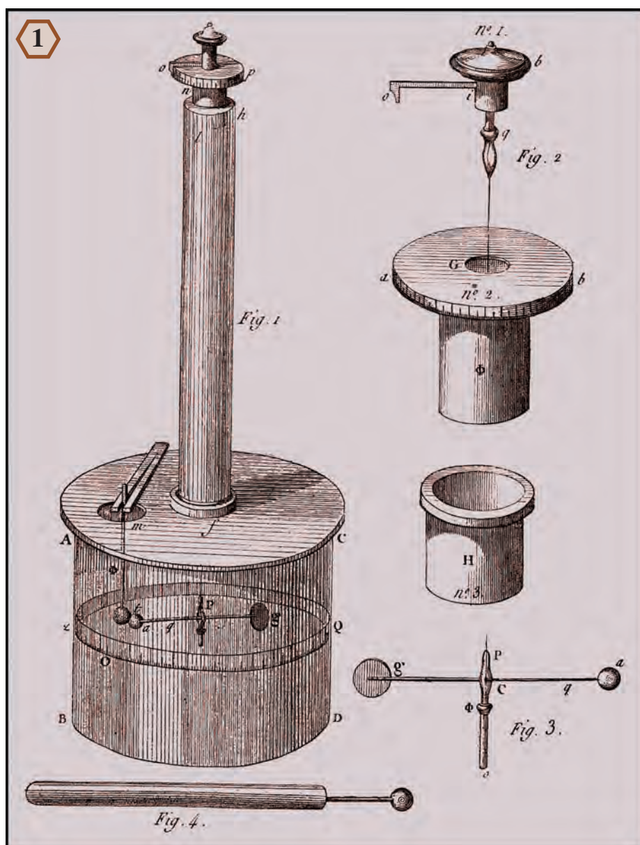
Illustration de la balance à torsion, utilisée par Coulomb pour mesurer les forces électriques de répulsion entre les charges semblables, tirée de son mémoire de 1785.
