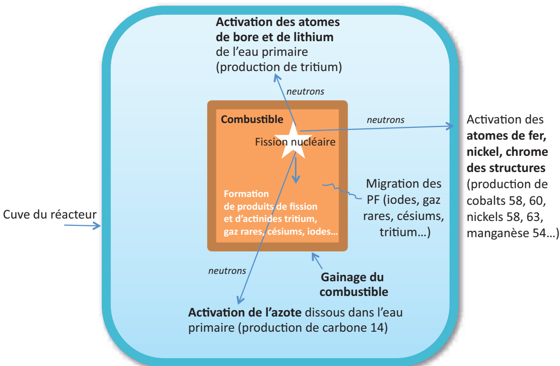
Fig. 3 → Produits de fission et les produits d'activation dans l'eau du circuit primaire
