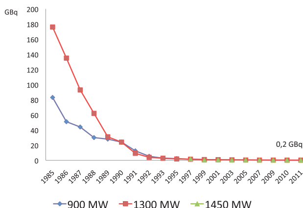
Fig. 13 → Réduction des rejets radioactifs liquides PF+PA, hors tritium et carbone 14 ; activité ramenée à une unité de production
