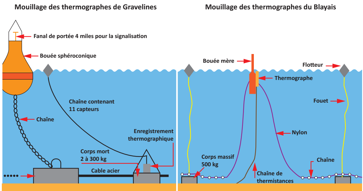
Fig. 4 → Schéma des thermographes
