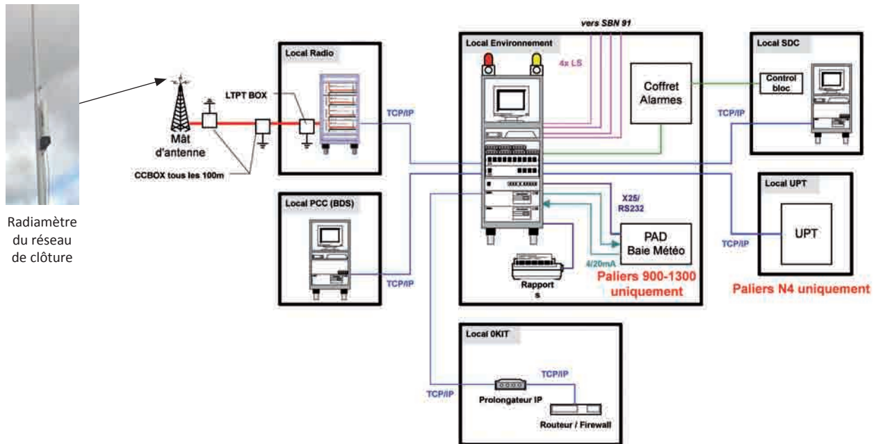
Fig.2 → Réseau de surveillance radiamétrique de clôture de site.
