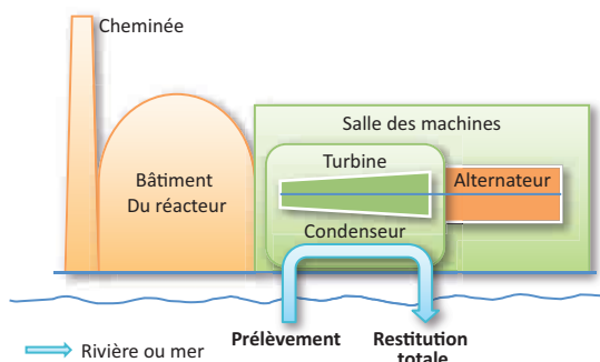
Fig. 5 → Circuit de refroidissement ouvert
