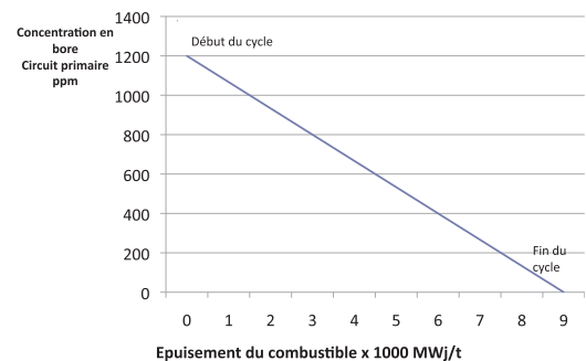
Fig. 13 → Évolution de la concentration en bore en fonction de l'épuisement du combustible
