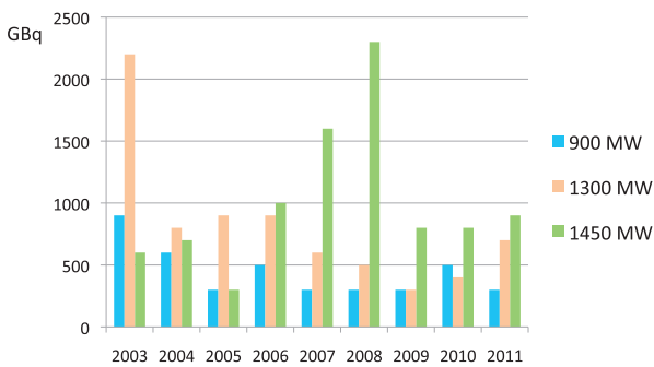
Fig. 6 → Rejet annuel moyen de gaz rares à la cheminée rapporté à un réacteur
